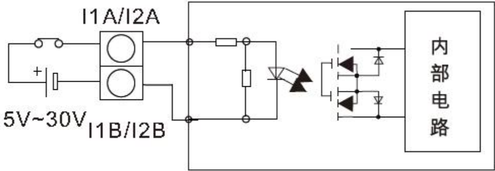
图 6. 触发输入电路连接示意图
